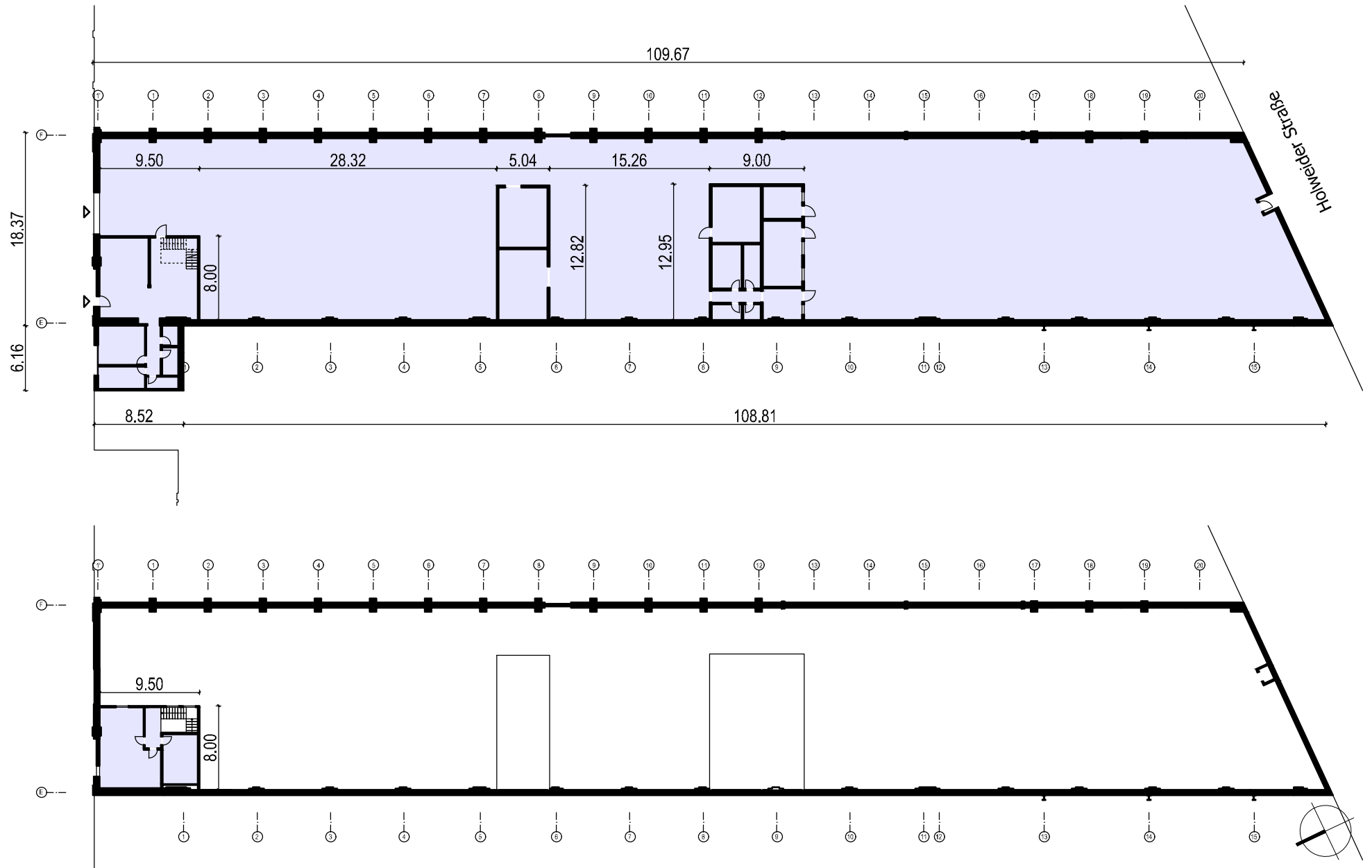
Grundriss Erdgeschoss und Obergeschoss
