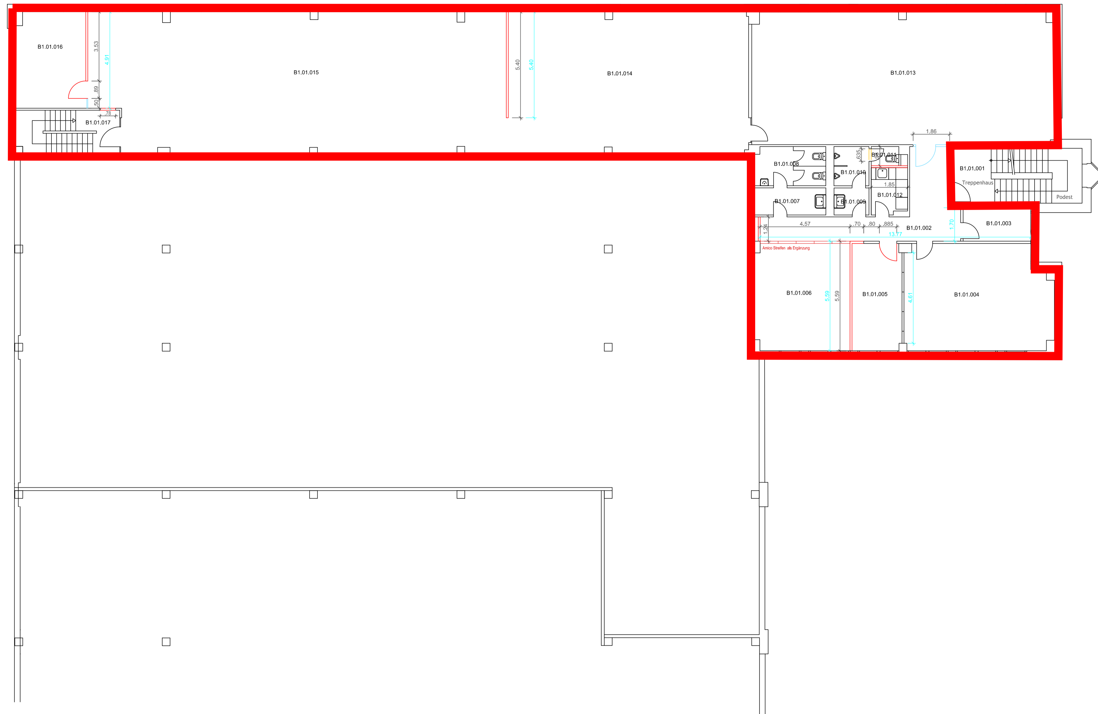
GRUNDRISS Bauteil B1— 1.0G M. 1:100
