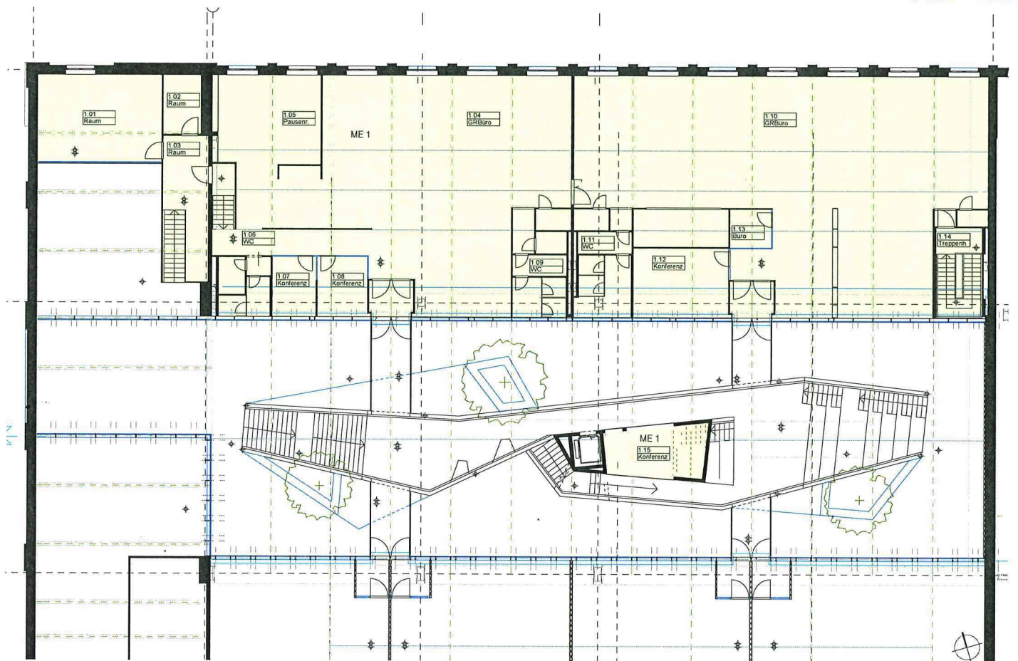
Grundriss Obergeschoss ME1
