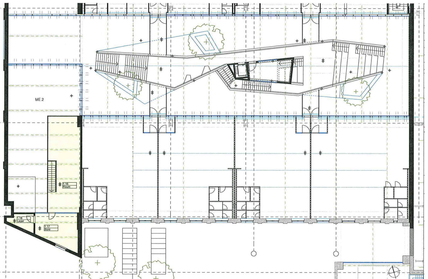
Grundriss Obergeschoss ME2
