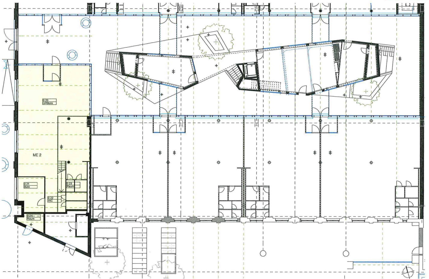
Grundriss Erdgeschoss ME2
